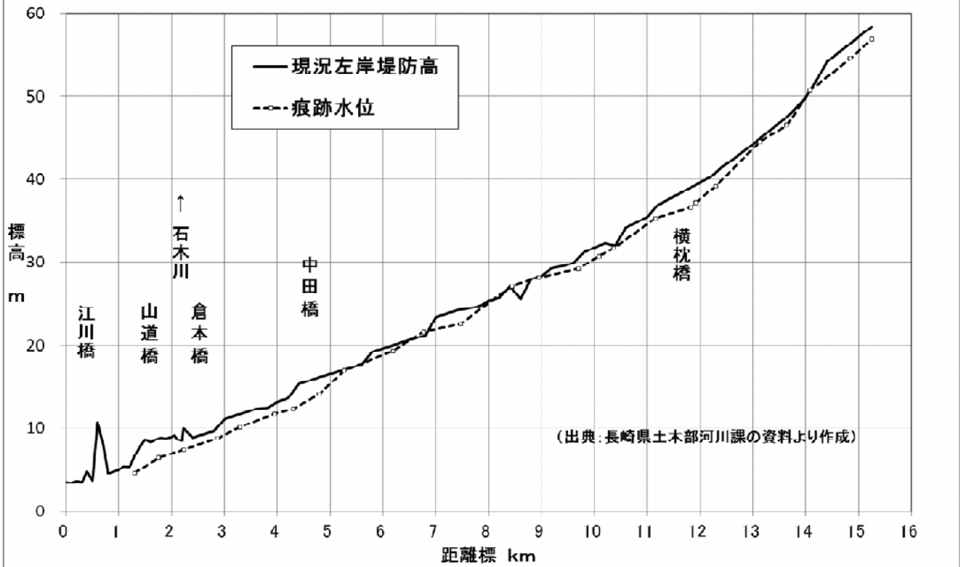
【図表3】(1) 川棚川 現況堤防高(左岸)と1990年7月洪水の最高痕跡水位
