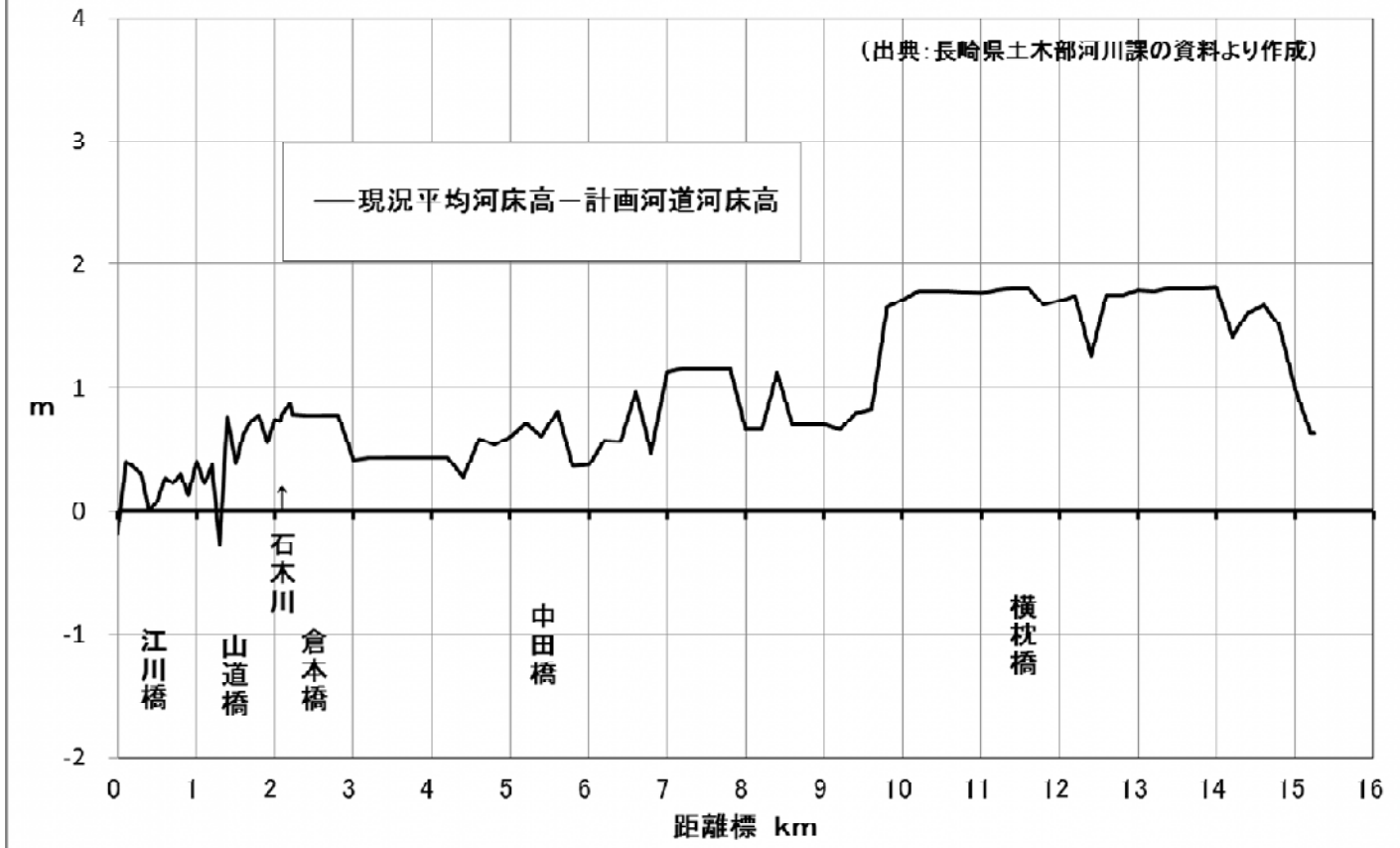
【図表4】川棚川 現況堤防高—計画河床高
